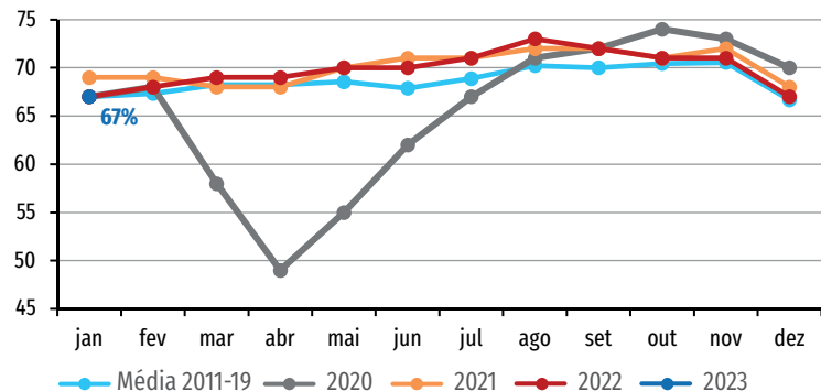
Utilização média da capacidade instalada Percentual (%)
