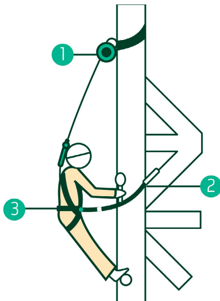
FIGURA 10 – EXEMPLO DE SISTEMA DE POSICIONAMENTO.
