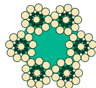
6X19 SEALE
