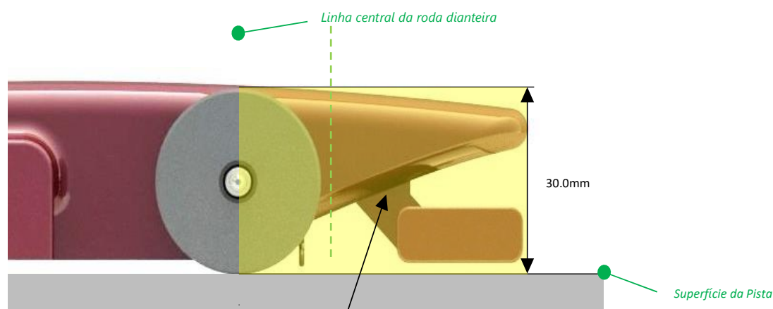
T10.3: Localização da asa dianteira e da estrutura de suporte da asa, destacado em amarelo
