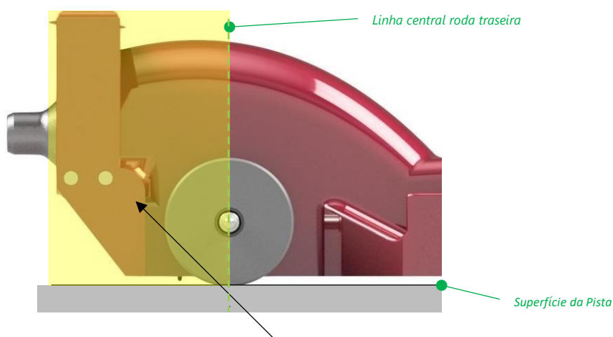
T9.3.2: Localização asa traseira e estrutura de suporte , destacado em amarelo
