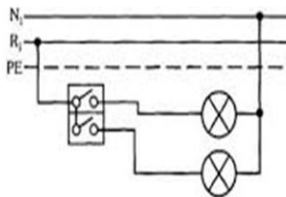
Diagrama multifilar:
