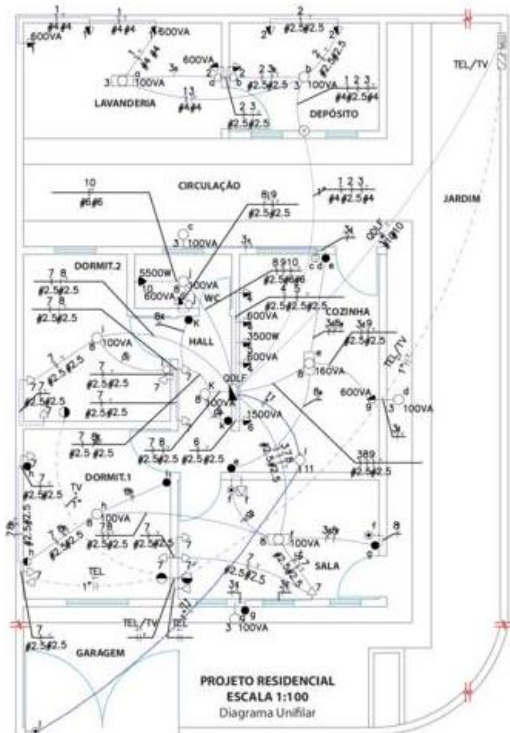
Figura 12 - Planta baixa final com todos os componentes, eletrodutos e condutores Fonte: SENAI-SP (2012)
