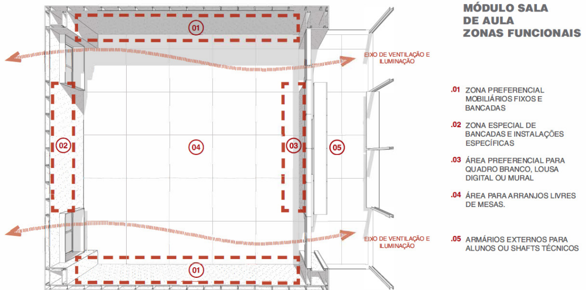
FIGURA 8 – Setorização da salade aula.
