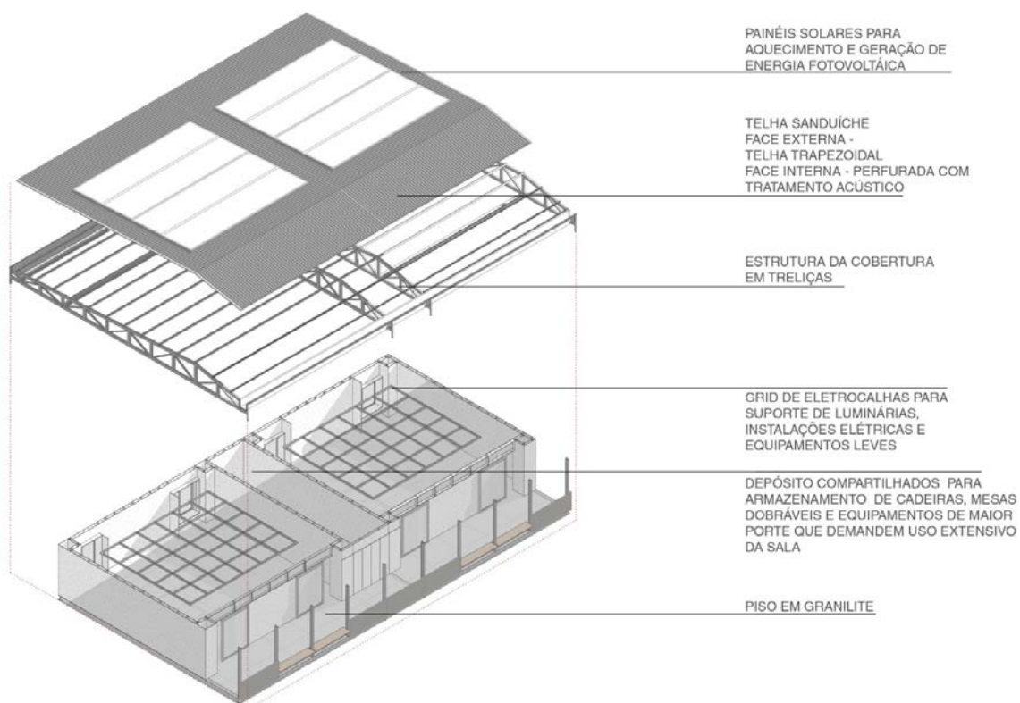
7. GRID DE FORRO E INSTALAÇÕES
