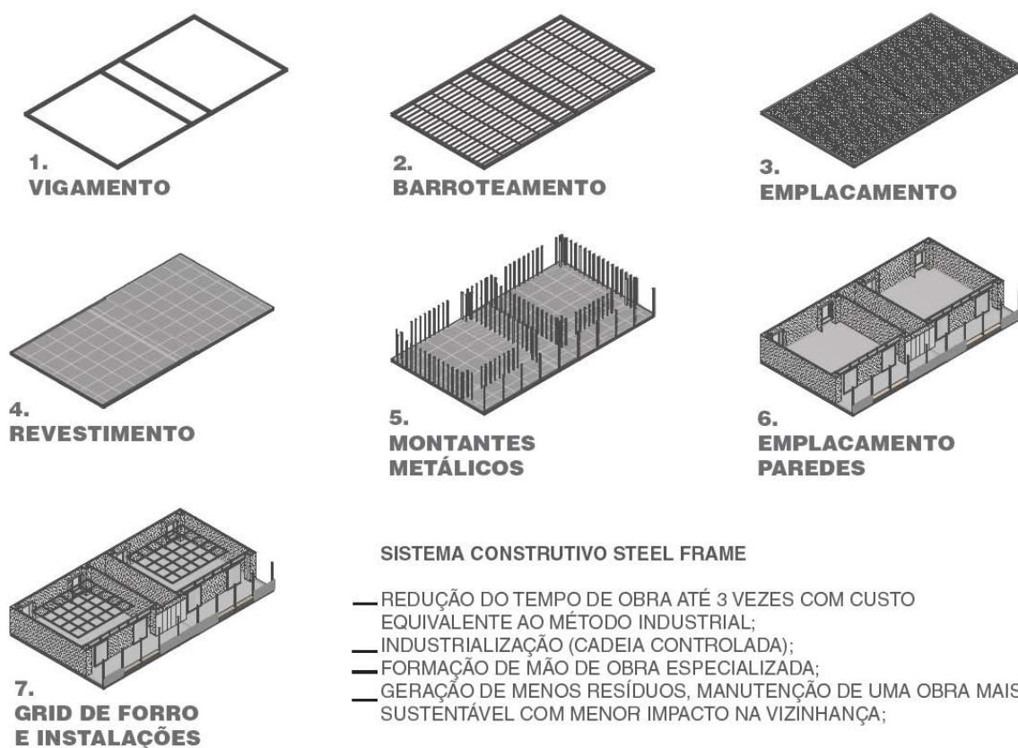
FIGURA 3 – Proposição de sistema construtivo Steel Frame.
